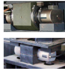
2 Messelement ABW-3 und ABW-4
